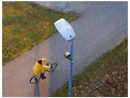
Leuchte Teceo mit Sensor zur Erkennung eines Radfahrers
